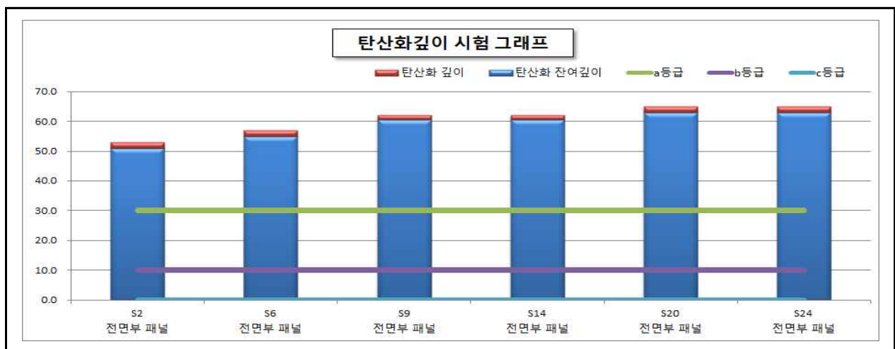
【그림 1.4.3】 탄산화 깊이 측정결과
